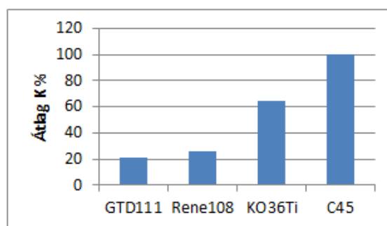
4. ábra. Forgácsolhatóság a kísérleti adatok szerint
